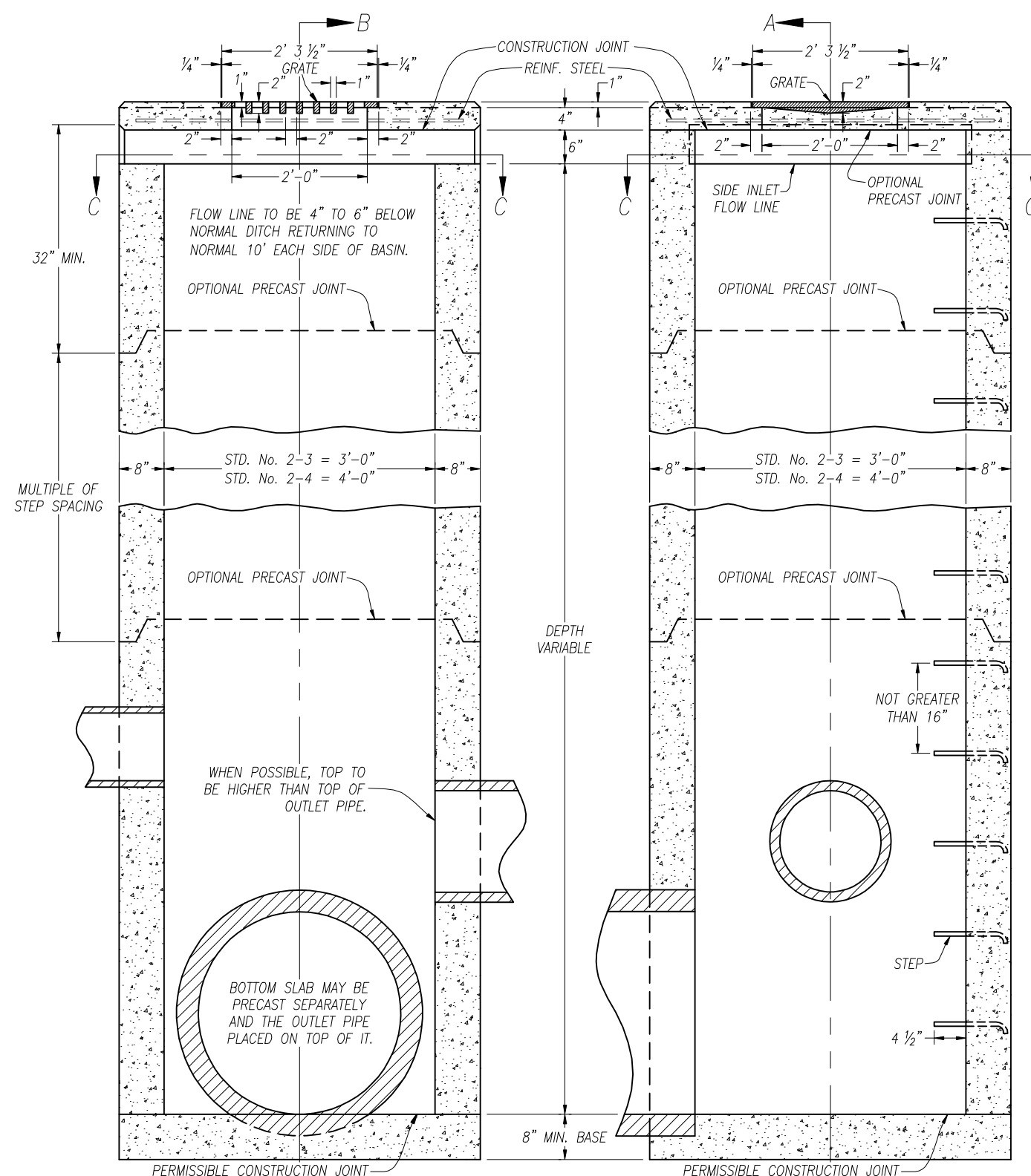
SECTION A-A
